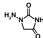
1-Aminohydantoin (AHD)
